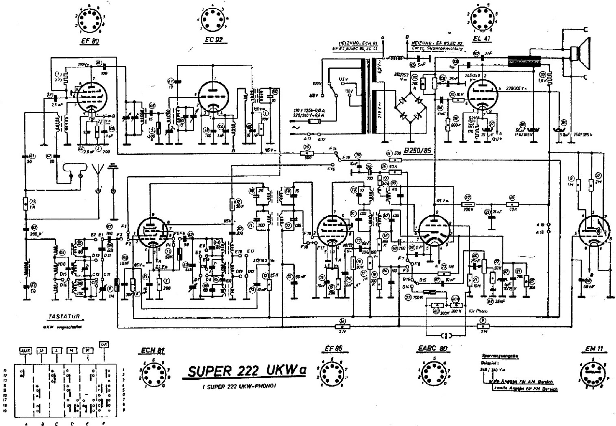
BRAUN (MAX BRAUN WERKE, FRANKFURT . MEIN). Mod. Super 222 UKW a. Apparecchio a modulazione di ampiezza e di frequenza; con cambio di gamma a tastiera. Media frequenza 460 kc/s.
